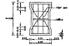
รายละเอียดเหล็กเสริมหางจรด
