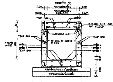
รายละเอียดเหล็กเสริมหางจรด
