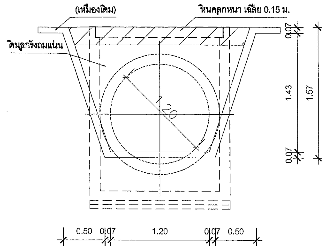
รูปตัดเหมือนเดิม (รื้อถอน)
