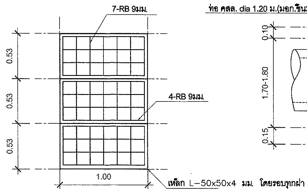
แปลนป้องกันน้ำ (ดูแบบขยาย) N/S
