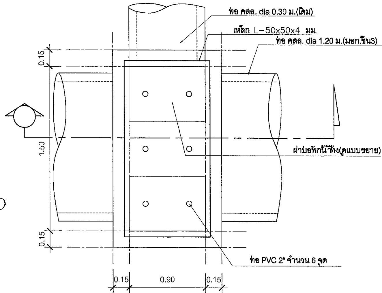
แปลนป้องกันน้ำ N/S
