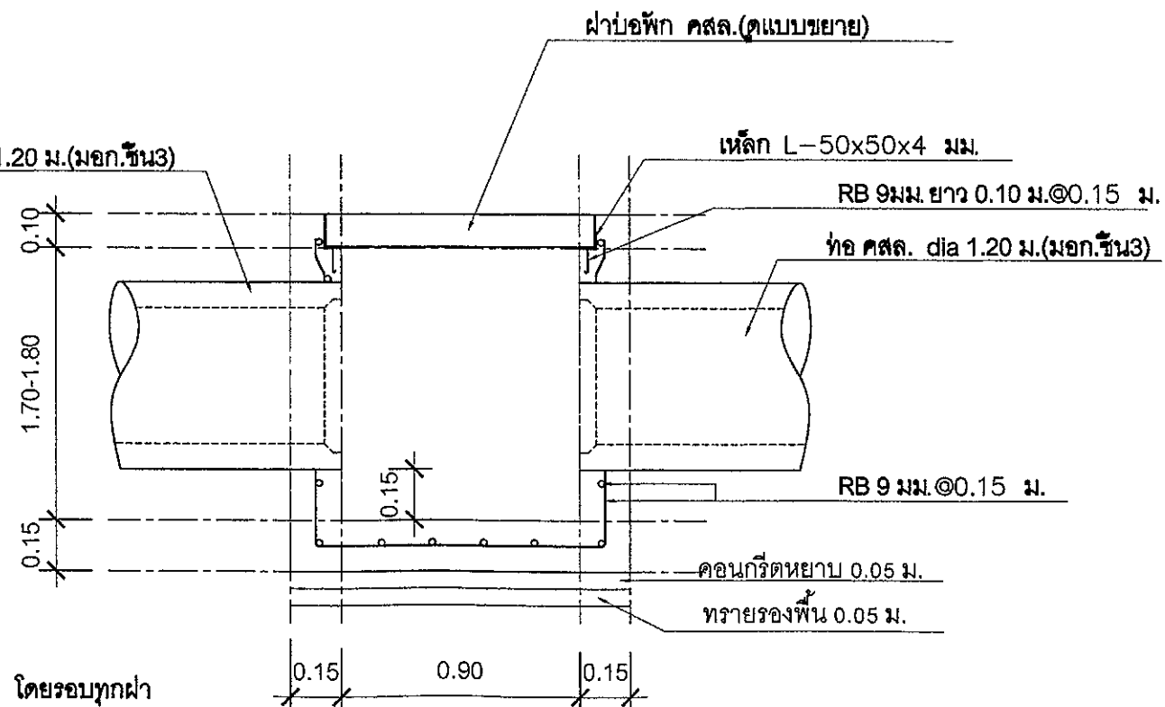
รูปตัดป้องกันน้ำ N/S
