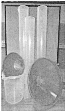
อุปกรณ์วัดอัตราการไหล และอัตราการเผาผลาญเชื้อเพลิง
